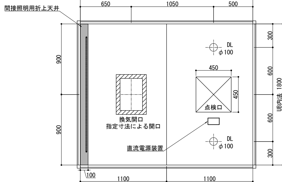
天井伏図
