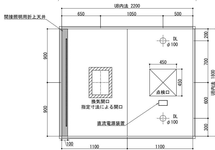
天井伏図
